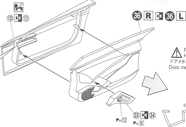
ドアサポートメタルステー Door suport metal stay
