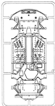
D部品 Tree D (16-1604-1)
