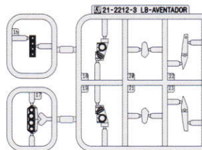
C 部品 (21-2212-3)
