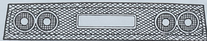
各部品取付原寸図
