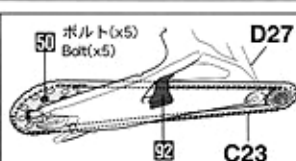
スイングアーム Swing arm
