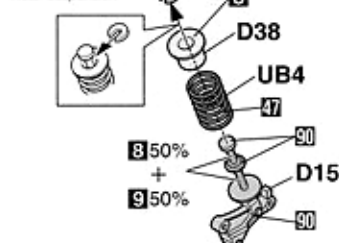
リヤサスペンション Rear suspension
