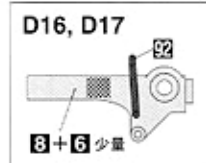
トレーリングアームの塗装 Trailing arm painting
