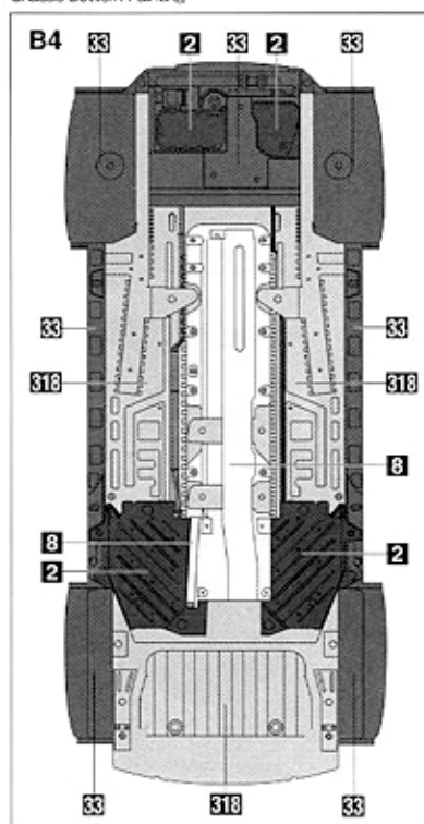
シャーシ下面の塗装 Chassis Bottom Painting
