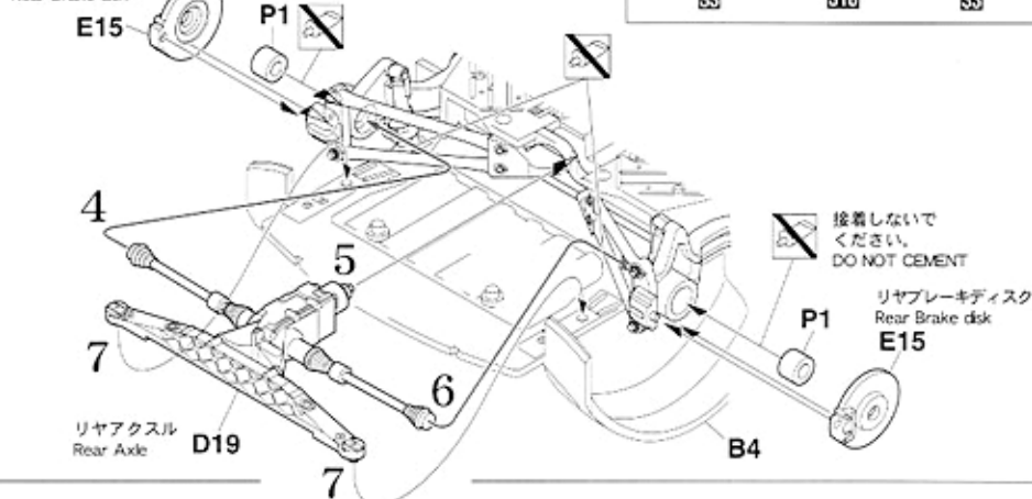
リヤブレーキディスク Rear Brake disk
